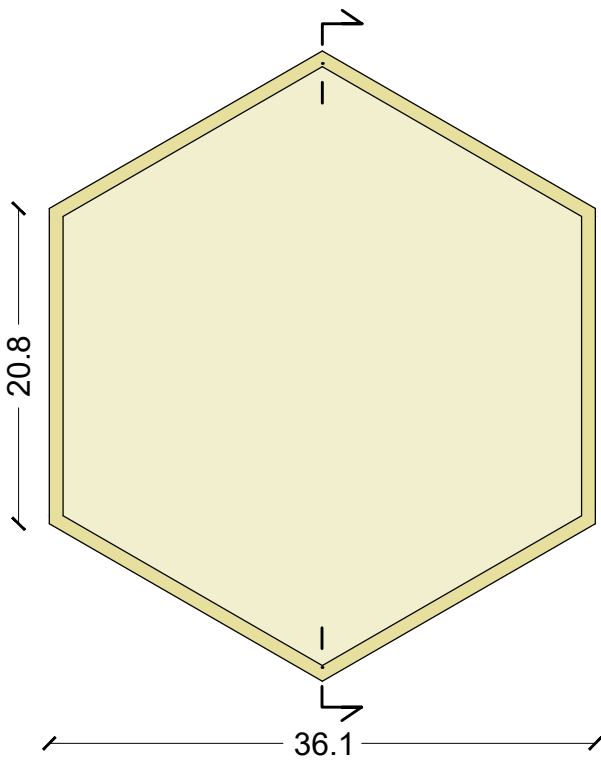
Fronte_scala 1:5
