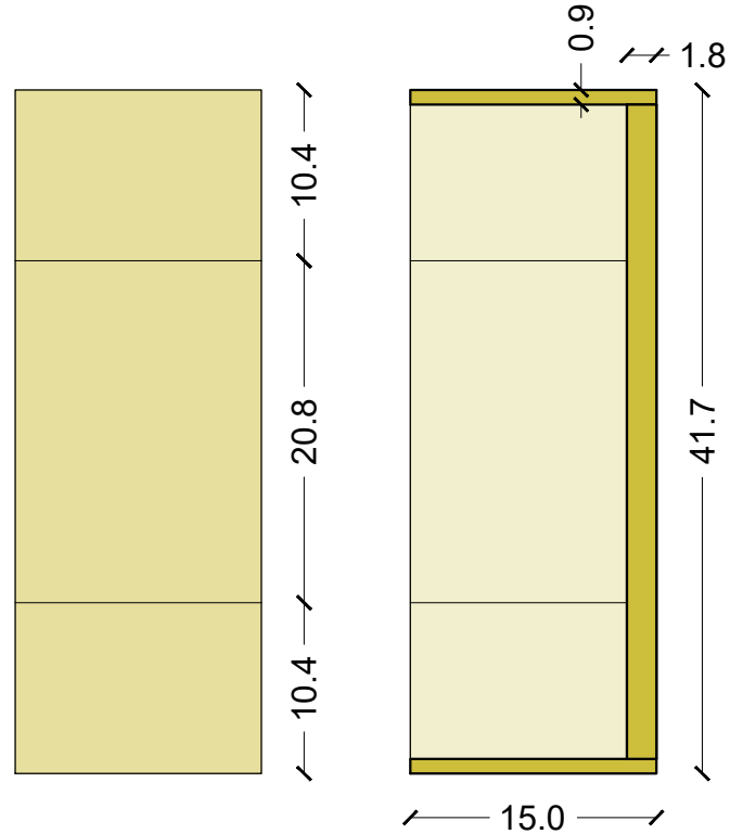
Visione laterale
